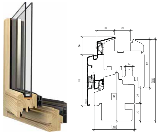
Naturo 68 RenoLine
