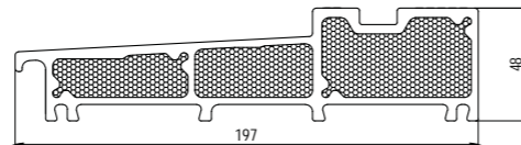
Schwelle 279110
