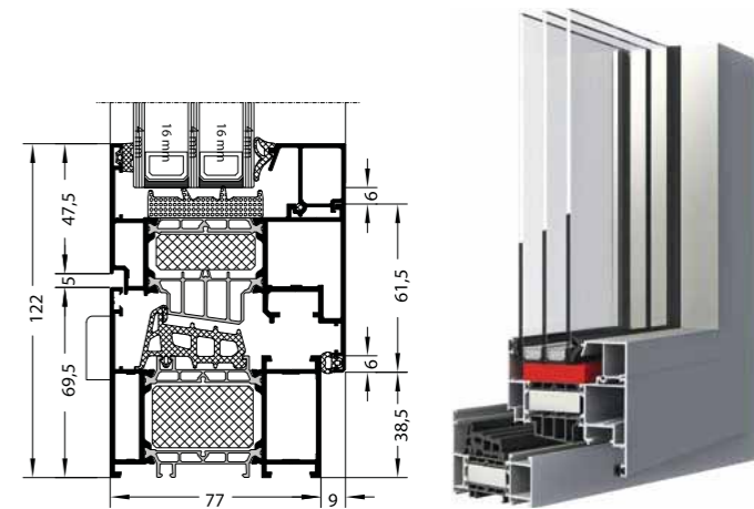
MB-86 Aero
